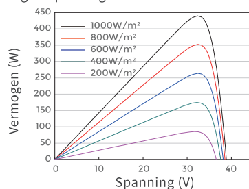
Vermogen-spanningscurve JAM54D41-440/LB
