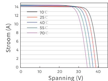
Stroom-spanningscurve JAM54D41-440/LB
