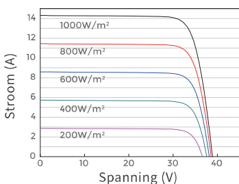
Stroom-spanningscurve JAM54D41-440/LB
